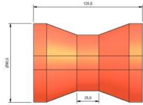
ROLLER 8
