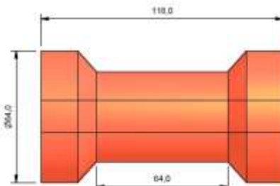
ROLLER 11
