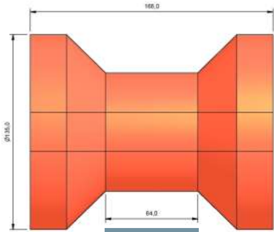
ROLLER 5
