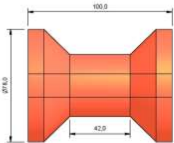
ROLLER 10
