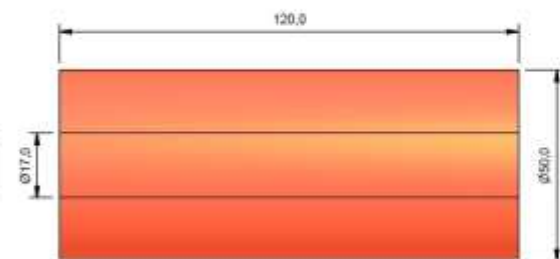
ROLLER 13
