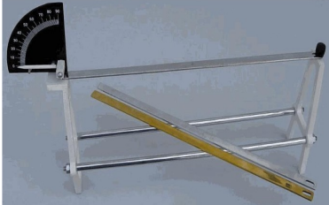
Linear expansion apparatus
